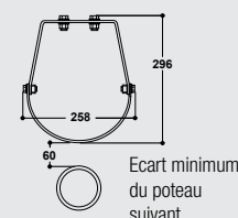
100.1239 + Accessoires pour circuit en boucle et résistance (images avec les vieux gabarits de perçage)
